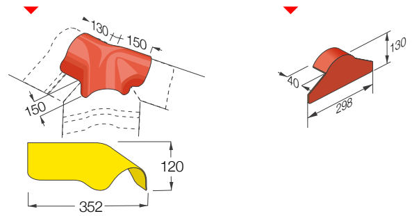
Endstück
