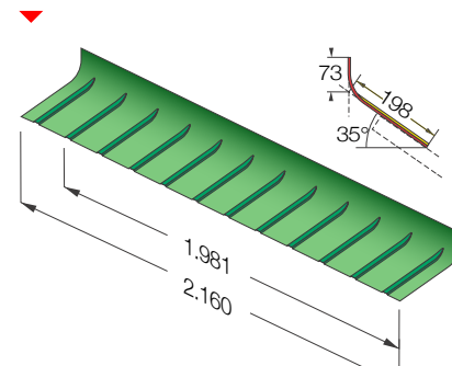
Maueranschlusstück
