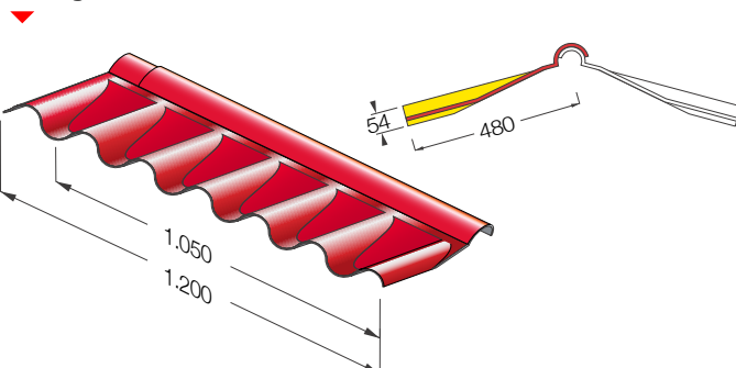
Pulldachabschluss
